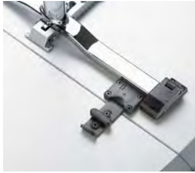
EHV1 Universalbeschlag für alle Tischplatten mit einer Plattenstärke von 30 mm
