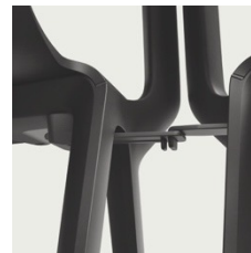
Ausziehbare Reihenverbindung
